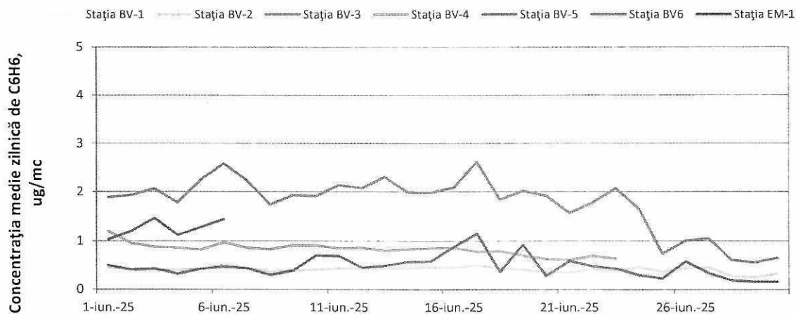
Figura 7. Evoluția concentrațiilor medii zilnice de benzen în luna iunie 2025
