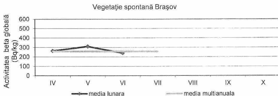
Fig. 28. Activitatea beta globală la 5 zile pentru vegetația spontană
