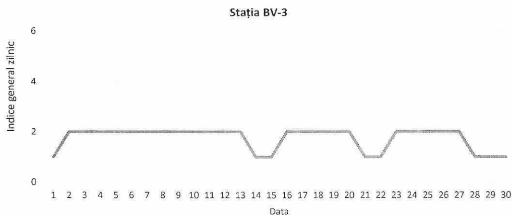
Figura 15. Evoluția indicelui general de calitate a aerului din stația BV-3
