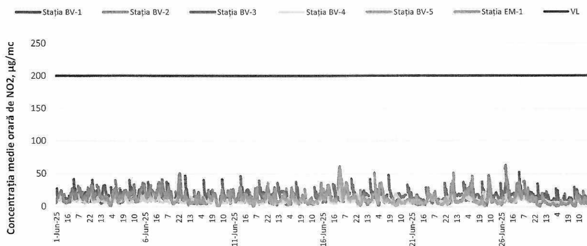
Figura 3. Concentrații medii orare de NO 2 în luna iunie 2025
