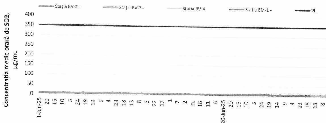
Figura 2. Evoluția mediilor orare de SO 2 în luna iunie 2025
