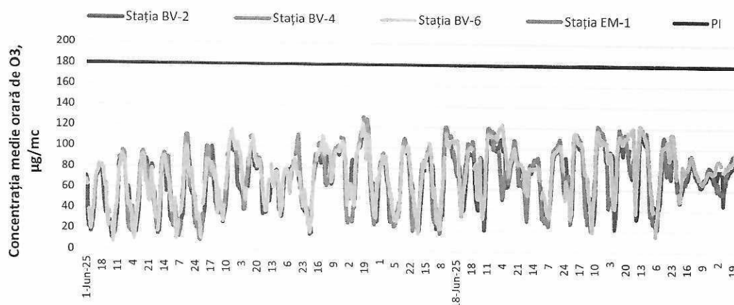
Figura 6. Evoluția concentrațiilor medii orare de O 3 în luna iunie 2025
