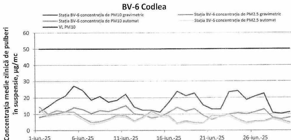
Figura 12. Evoluția concentrațiilor medii zilnice de PM10 gravimetric și automat și PM2,5 gravimetric și automat în stația de fond urban BV-6 în luna iunie 2025
