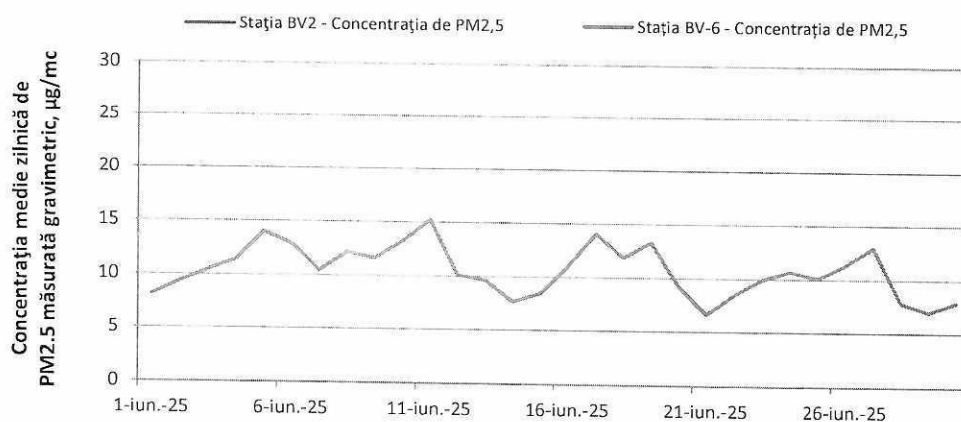
Figura 11. Evoluția concentrațiilor medii zilnice de PM 2,5 (gravimetric) în luna iunie 2025
