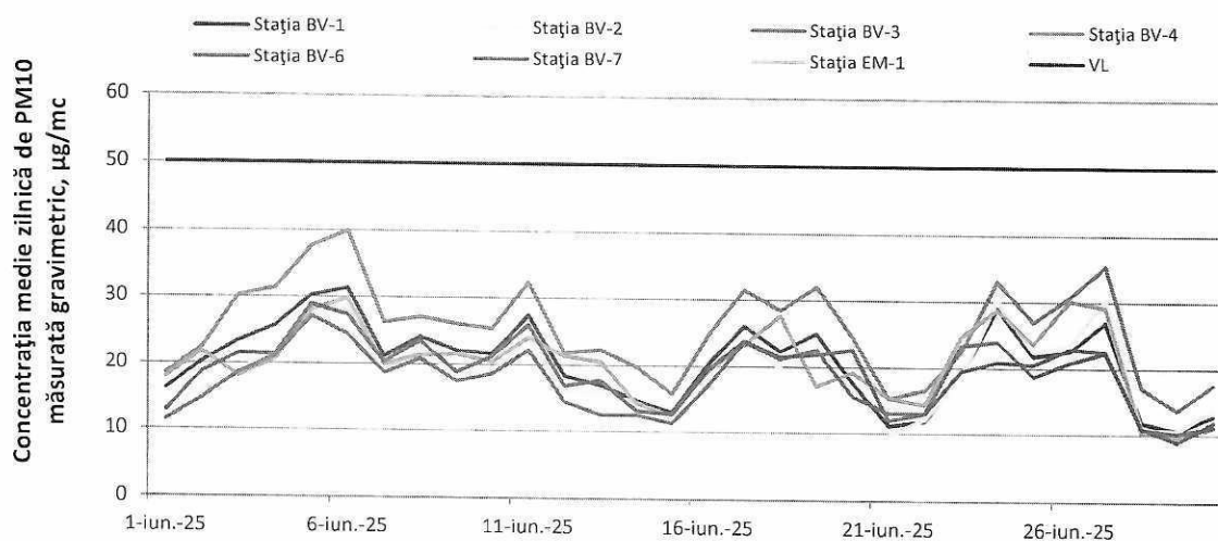
Figura 8. Evoluția concentrațiilor medii zilnice de PM10 (gravimetric) în luna iunie 2025
