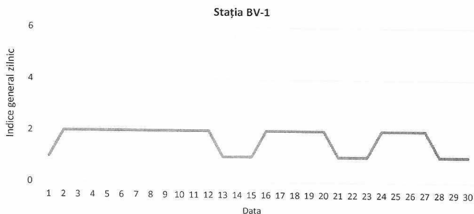
Figura 13. Evoluția indicelui general de calitate a aerului din stația BV-1
