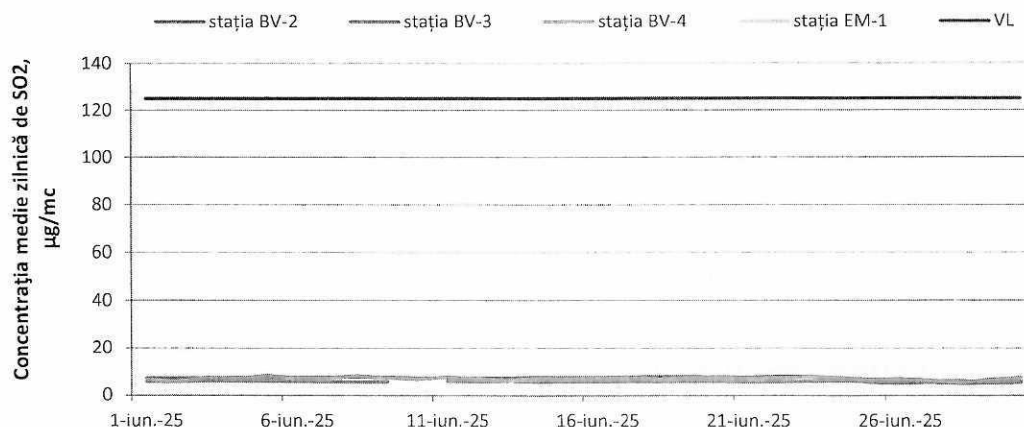
Figura 1. Evoluția mediilor zilnice de SO 2 în luna iunie 2025
