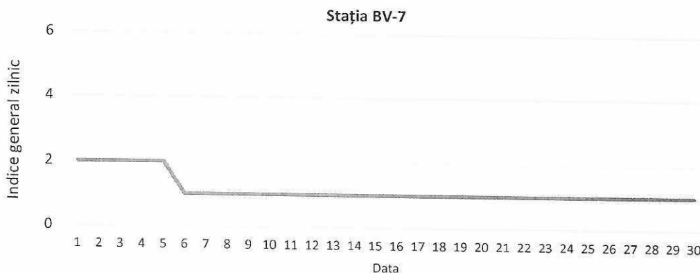
Figura 19. Evoluția indicelui general de calitate aerului din stația BV-7
