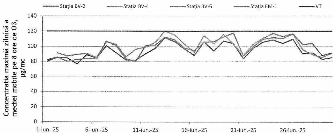
Figura 5. Evoluția concentrațiilor maximelor zilnice ale mediilor mobile pe 8 ore de O 3 în luna iunie 2025
