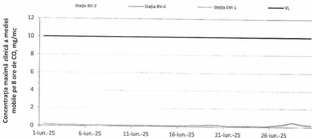
Figura 4. Concentrația maximă a mediei mobile pe 8 ore de CO în luna iunie 2025
