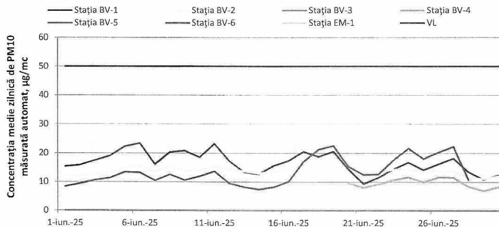
Figura 10. Evoluția concentrațiilor medii zilnice de PM 10 automat în luna iunie 2025
