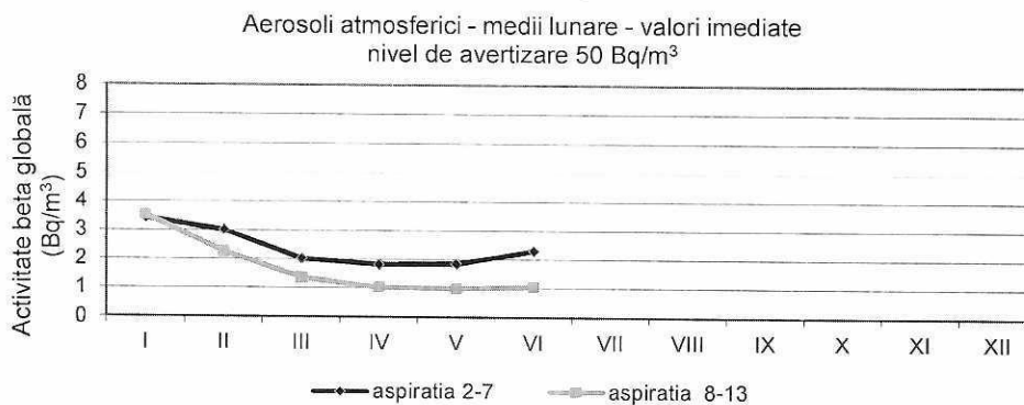
Figura 20. Activitatea beta globală pentru aerosoli atmosferici
