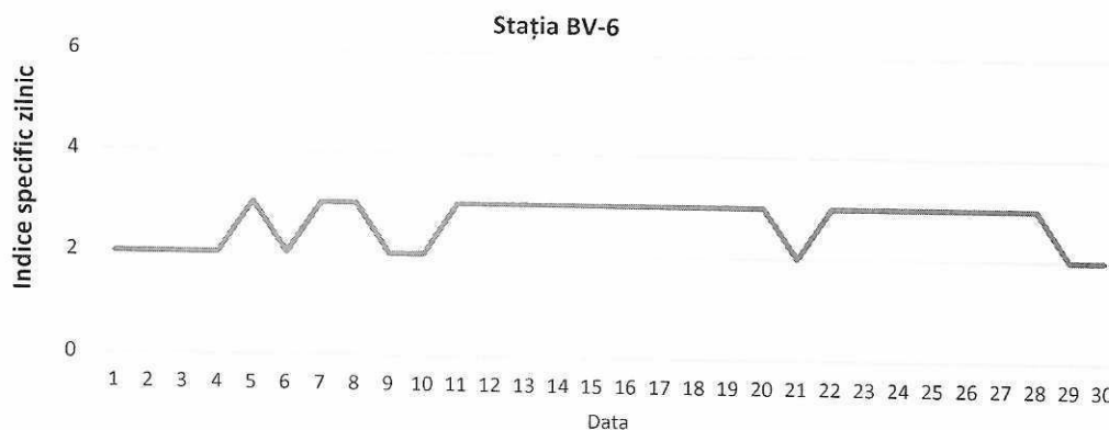
Figura 18. Evoluția indicelui general de calitate aerului din stația BV-6
