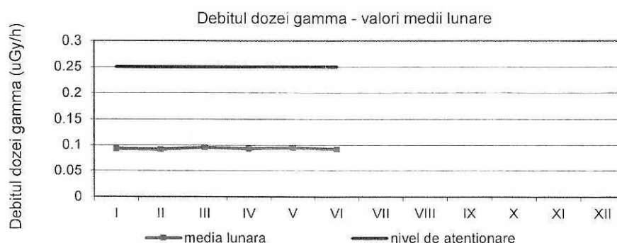
Figura 22. Debitul dozei gamma
